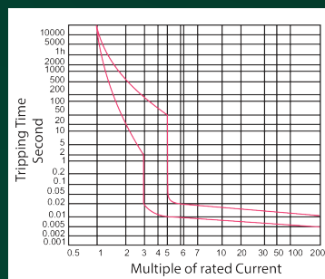
منحنی مشخصه B (روشنایی)
