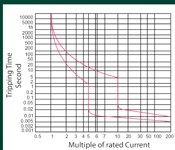
منحنی مشخصه C (موتوری)
