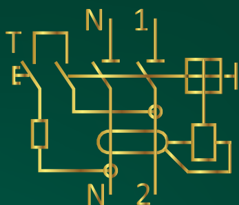
دیاگرام فنی (دوپل)
