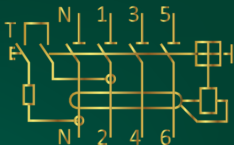
دیاگرام فنی (چهارپل)
